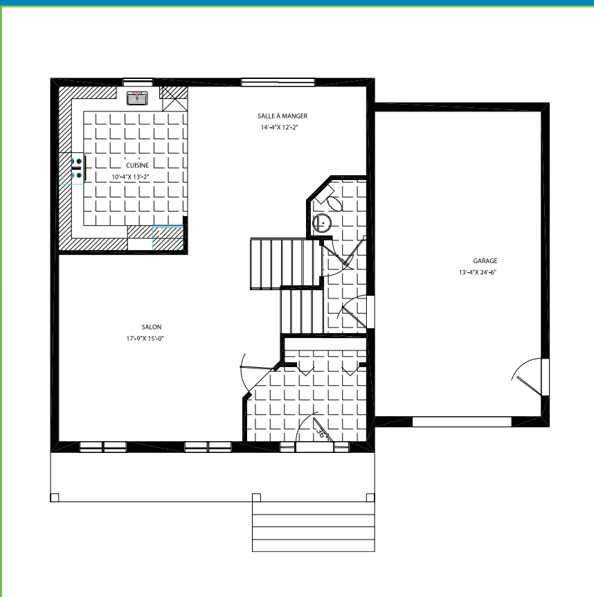
Rez-de-chaussée
